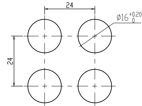
Install size / Bohrbild
