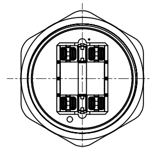
Schaltkreis
