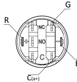
Schaltkreis
