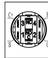
PIN Anordnung
