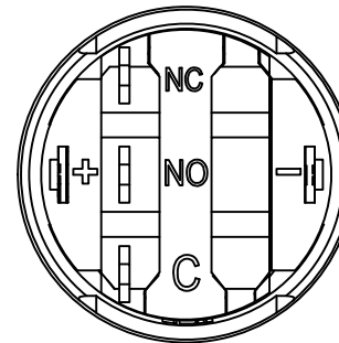
Schaltkreis
