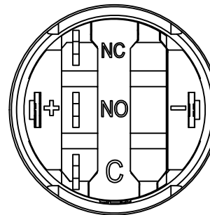
Schaltkreis
